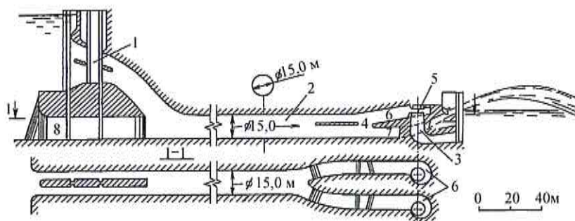
1 – совмещенный водоприемник гидроагрегатов и глубинного водосброса; 2 – подводящий туннель; 3 – глубинный водосброс; 4 – отверстия в разделительных диафрагмах; 5 – турбинный блок; 6 – подводящий тракт гидроагрегатов; 7 – глубинный водосброс; 8 – водоприемник строительного туннеля
