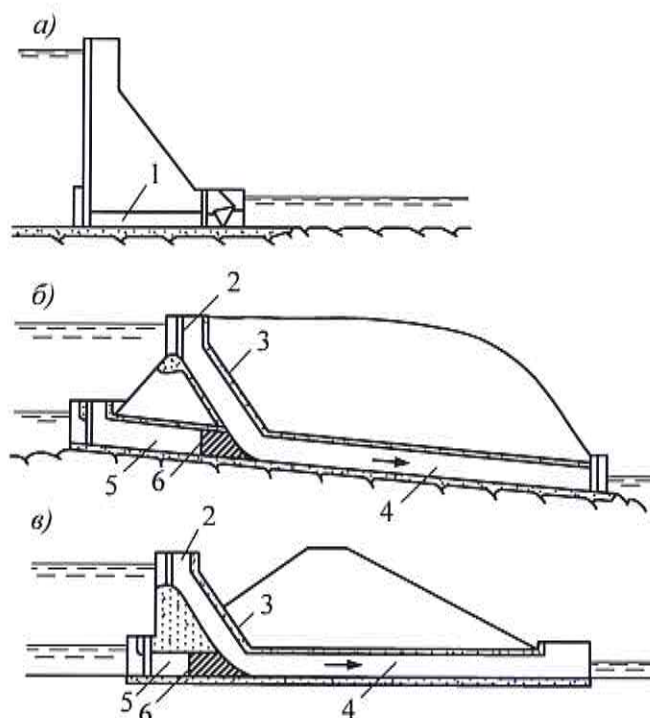
а) – донный водосброс в бетонной плотине; б) – туннельный водосброс; в) – трубчатый водосброс под грунтовой плотиной; 1 – строительно-эксплуатационный водосброс; 2 – входная часть эксплуатационного водосброса; 3 – сопрягающий участок эксплуатационного водосброса; 4 – отводящий участок; 5 – участок строительного водосброса; 6 – пробка
