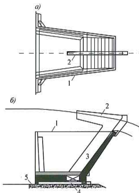
а) – план; б) – продольный разрез; 1 – гребень лабиринтного водослива; 2 – гребень водоприемника рабочей камеры; 3 – водовод рабочей камеры; 4 – рабочая камера; 5 – гребень плотины (порог затвора)
