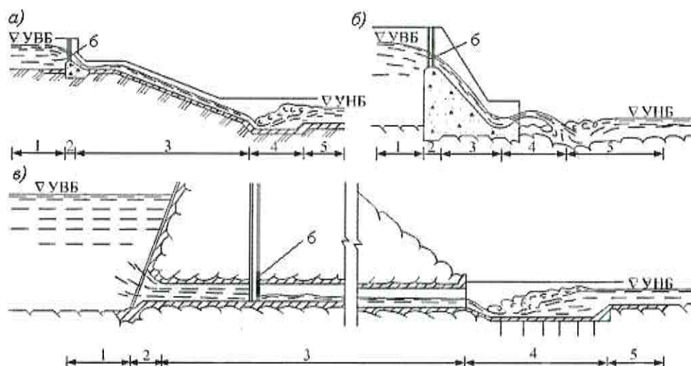
а) – открытый береговой водосброс; б) – открытый русловой водосброс в виде водосливной плотины с высоким порогом; в) – закрытый туннельный водосброс
