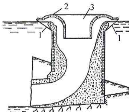
1 – входные отверстия; 2 – капор; 3 – отверстия для сброса мусора
