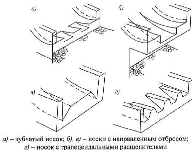
Рисунок – 38 Различные типы носков-трамплинов
