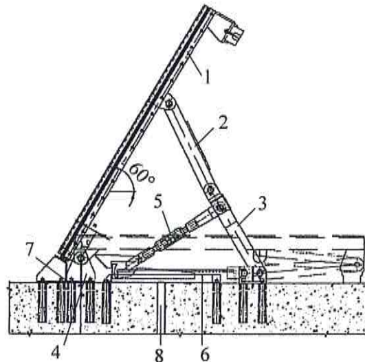
1 – полотнище затвора; 2,3 – звенья опорной штанги; 4 – шарнир затвора; 5 – толкатель; 6 – рабочая камера; 7 – гребень плотины (порог затвора); 8 – водовод от водоприемника
