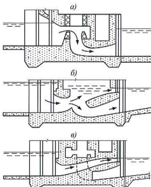
а) – через турбинный тракт; б) – через недостроенные донные водосбросы совмещенной ГЭС и отсасывающую трубу; в) – через донные водосбросы совмещенной ГЭС
