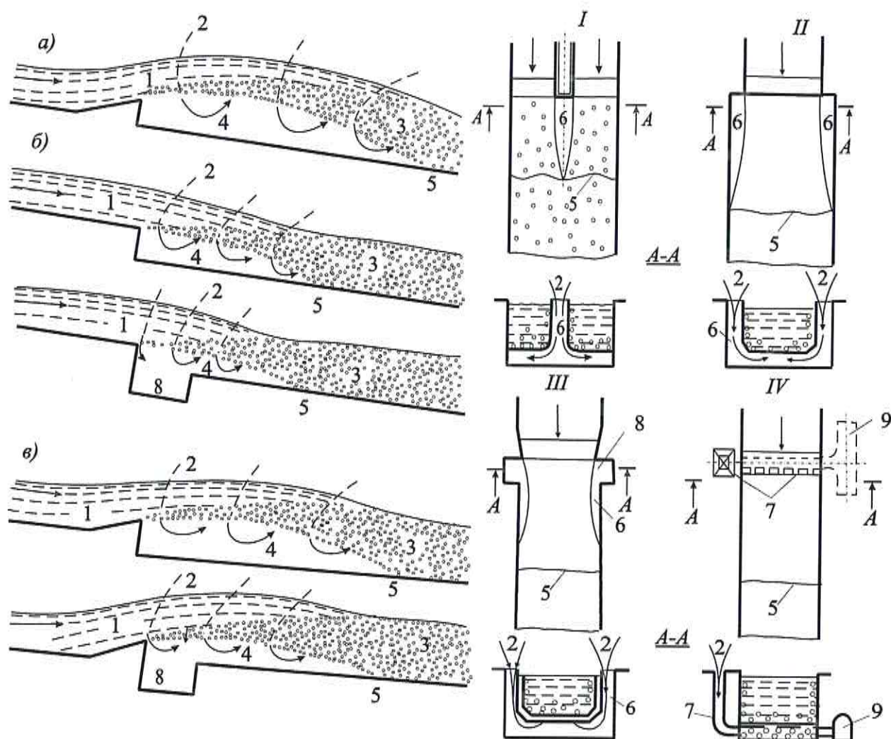
Продольные разрезы по оси азраторов: а) –трамплинный; б) и в) – ступенчатый и комбинированный без воздухоподводящего (азрационного) паз и с воздухоподводящим пазом на дне; Схемы подвода воздуха : I – полостная за бычком; II – полостная за ступенчатым или трамплинным отклонителем; III – с боковым воздухоподводящим пазом; IV – канальная; 1 – неаэрированный поток; 2 – подвод воздуха; 3 – водовоздушная смесь; 4 – подструйная полость; 5 – граница в конце подструйной полости; 6 – воздухоподводящая полость; 7 – воздуховод; 8 – воздухоподводящий паз; 9 – воздухоподводящая галерея
