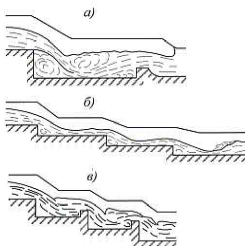
Рисунок 17 – Схемы перепадов
