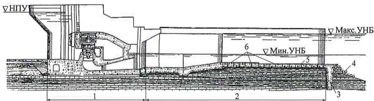
1 – здание ГЭС; 2 – крепление (водобой и рисберма); 3 – концевой зуб; 4 – защитная каменная наброска; 5 – горизонтальный дренаж; 6 – дренажные колодцы
