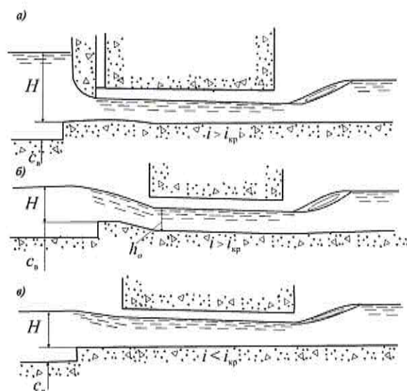
а – с забальной стенкой; б – с водосливным порогом; в – в виде водослива без порога
