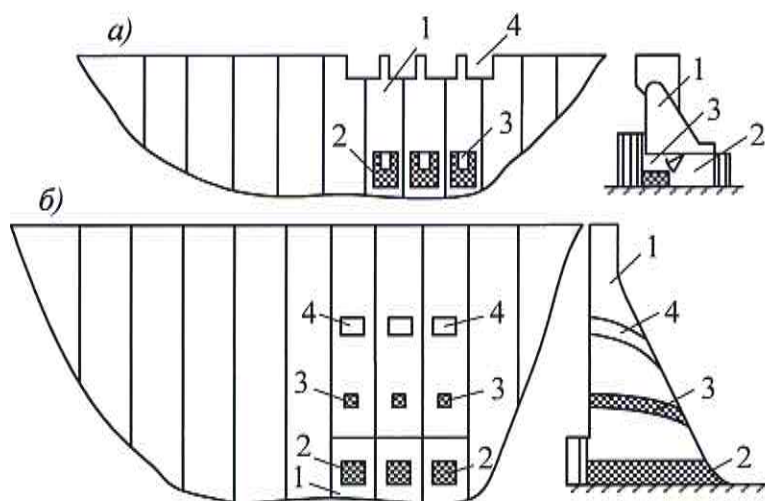
а – плотина с эксплуатационными поверхностными водосбросами; б) – плотина с эксплуатационными глубинными водосбросами; 1 – тело плотины; 2 – донные водосбросы I яруса; 3 – донные водосбросы II яруса; 4 – эксплуатационные водосбросы
